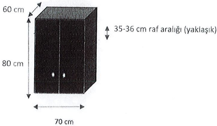
3.8. Dolap-80x70x60 cm -(Beyaz)
